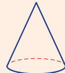
Cone
